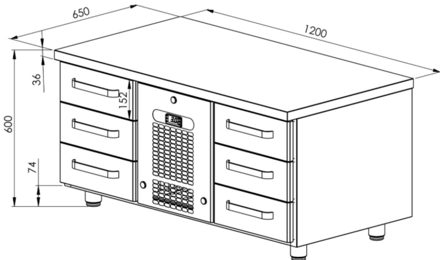
Måttskiss
