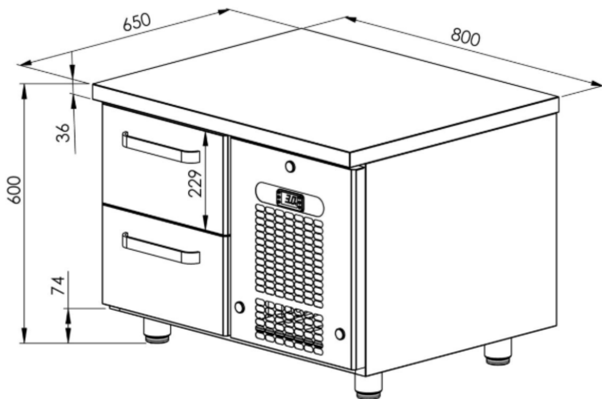
Måttskiss
