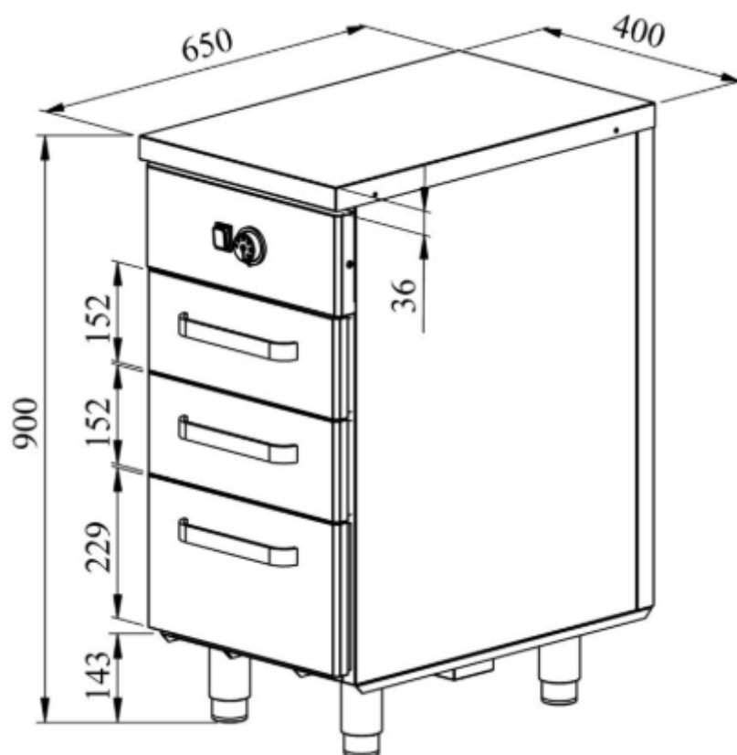
Måttskiss
