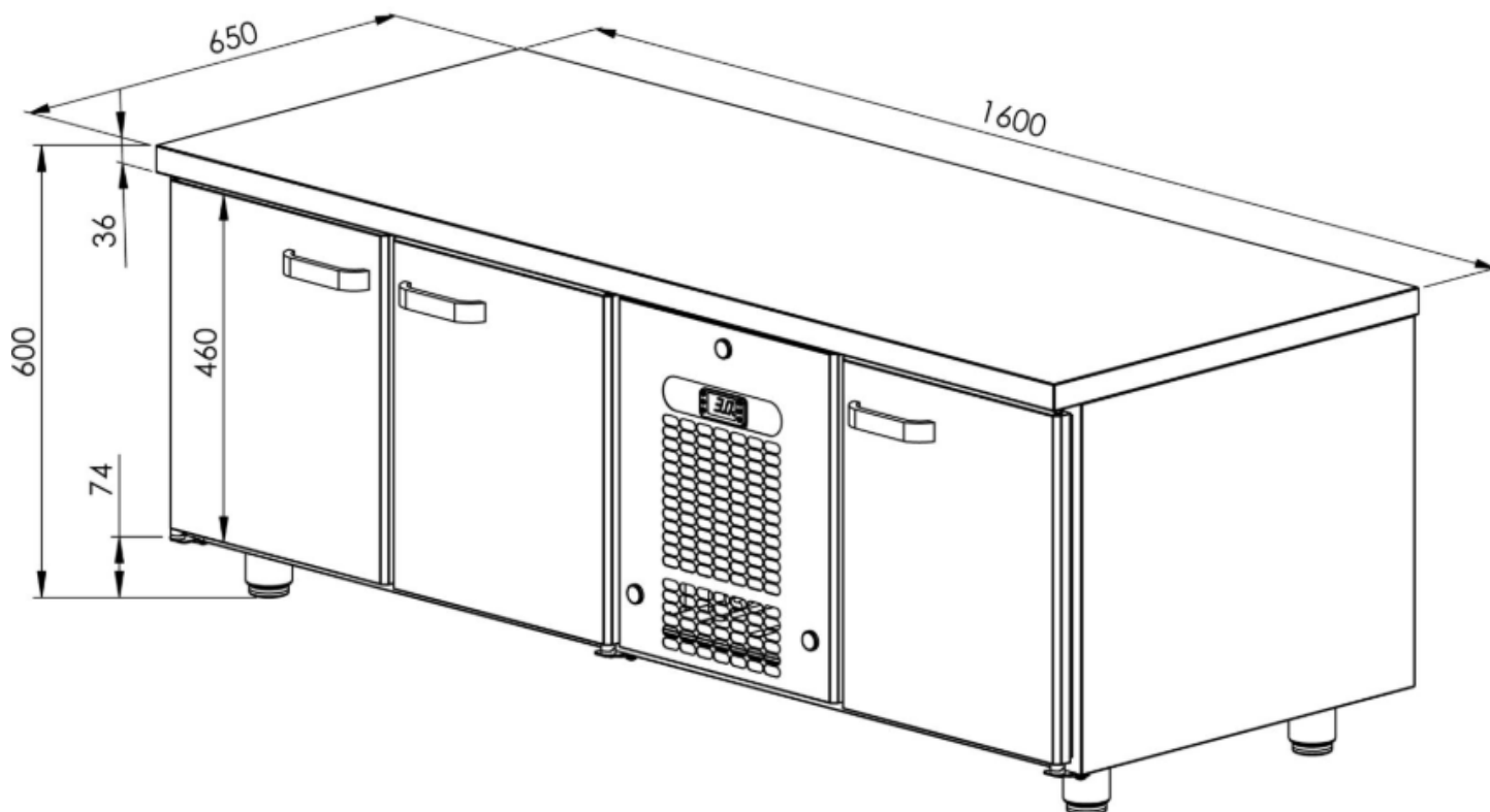
Måttskiss
