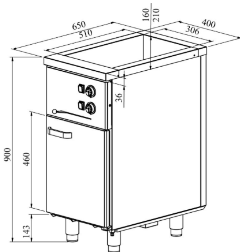
Måttskiss
