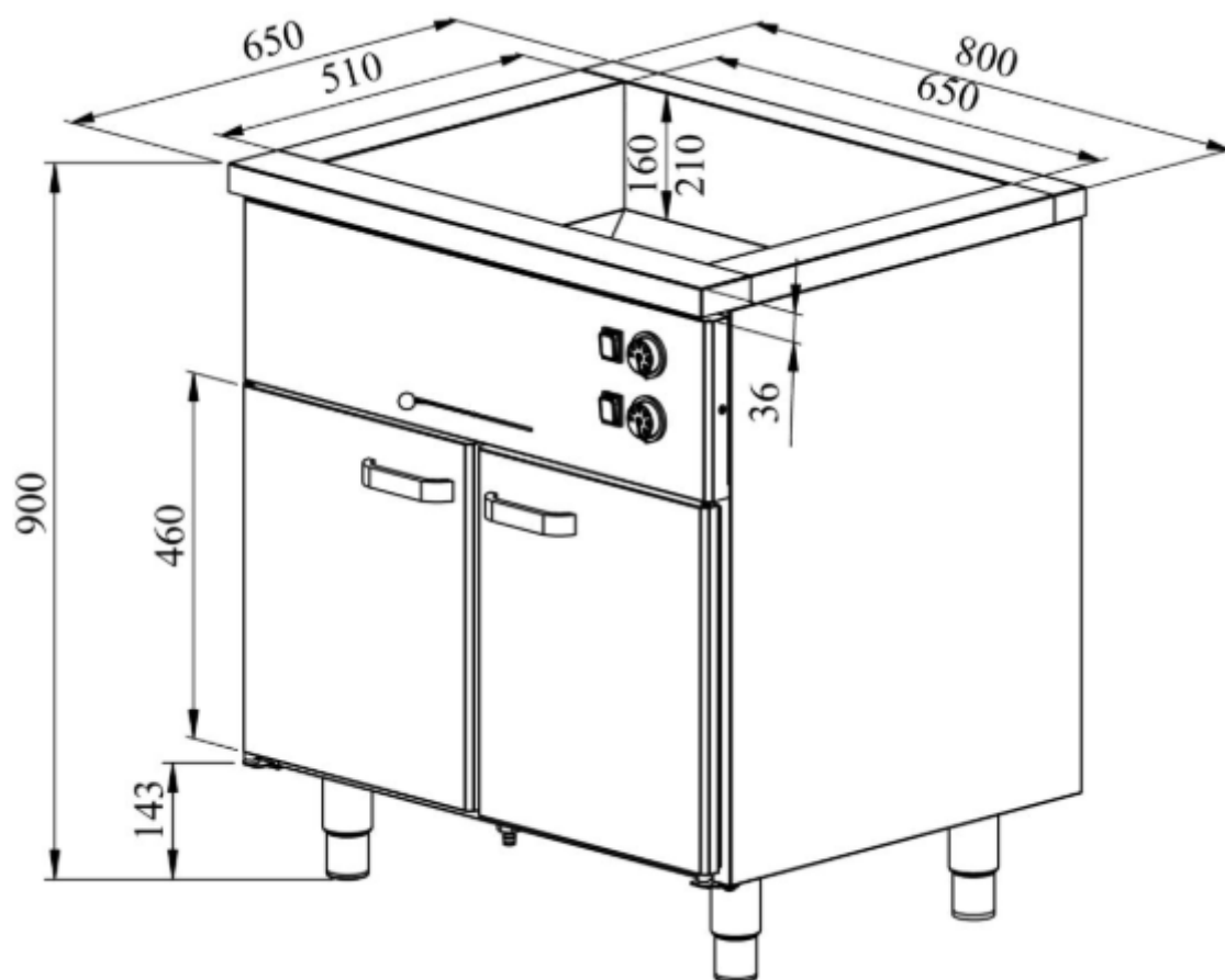
Måttskiss
