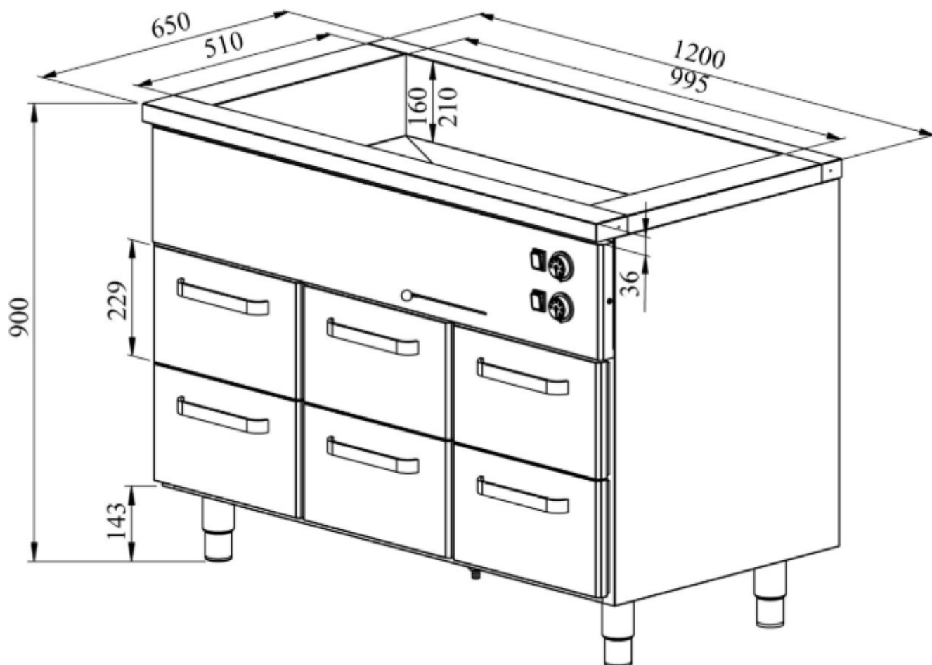
Måttskiss
