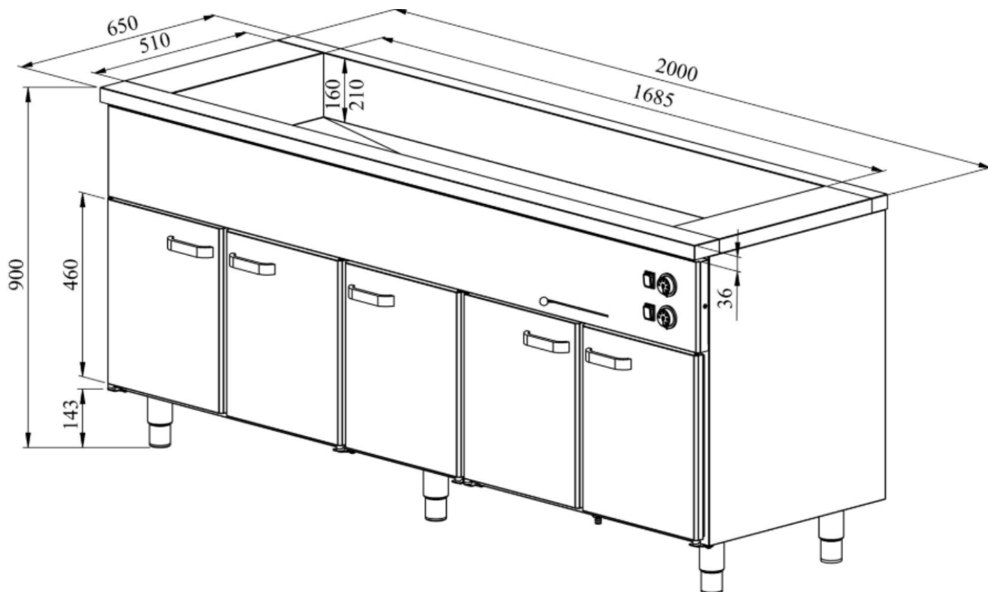
Måttskiss
