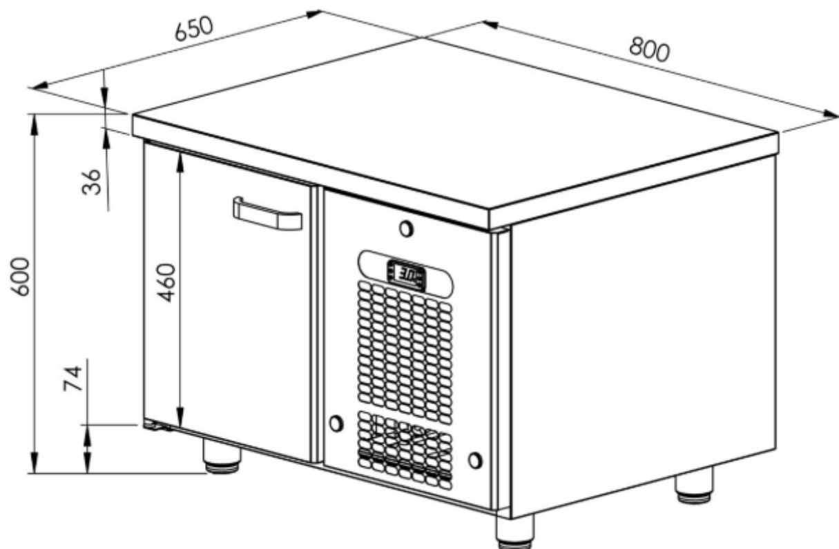
Måttskiss
